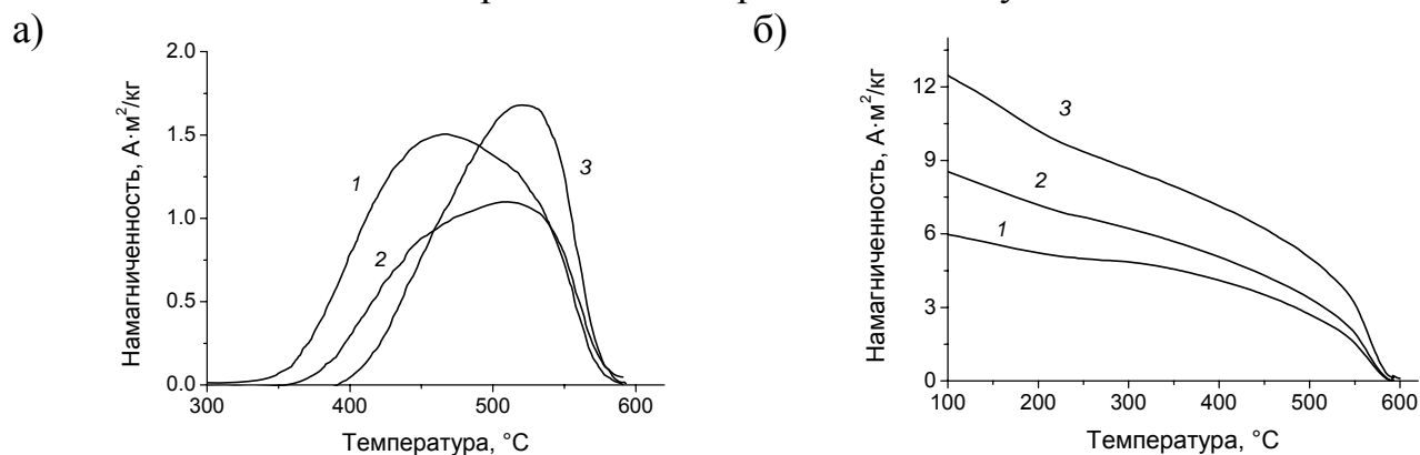
Рис. 1. Зависимость удельной намагниченности от температуры в процессе прокаливания в потоке аргона (а) и термомангнитная зависимость после прокаливания (б) (1 – Fe/Syb, 2 – Fe1K/Syb и 3 – Fe2K/Syb).
