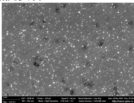
Рис.1 SEM-изображение осажденного ансамбля наночастиц состава «Со-Си» со средним размером 80 нм на поверхности кремния.
