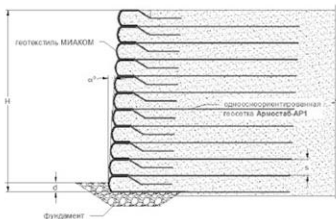
Рисунок 3 Подпорная стенка, армированная геотекстилем
