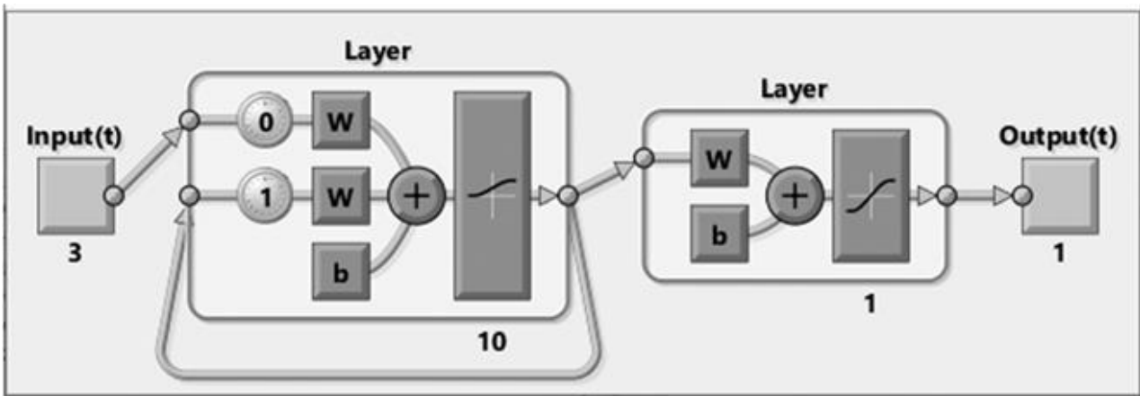
Рисунок 2. Модель на базе рекуррентной сети
