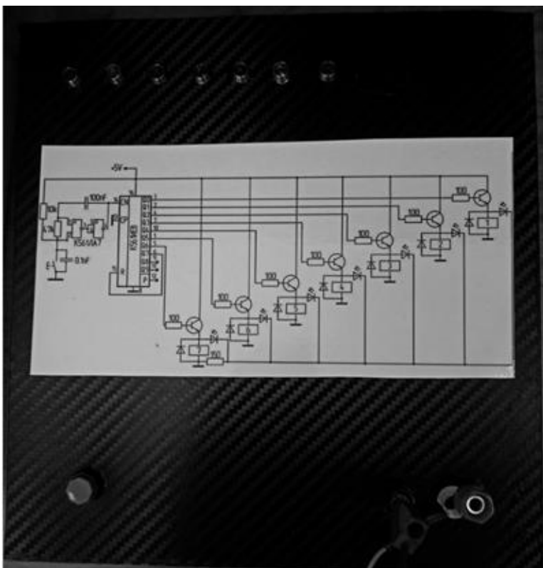
Рисунок 1–Внешний вид лабораторного макета
