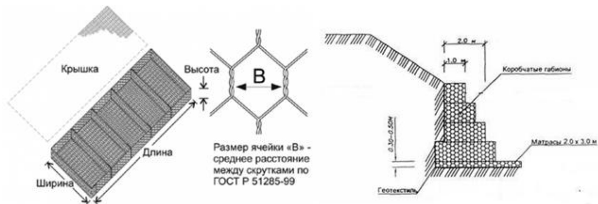
Рисунок 1 Подпорная стенка из коробчатых габионных конструкций
