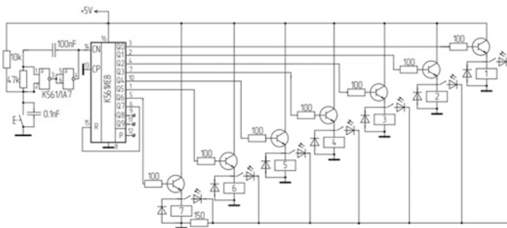
Рисунок 3 – Принципиальная электрическая схема установки
