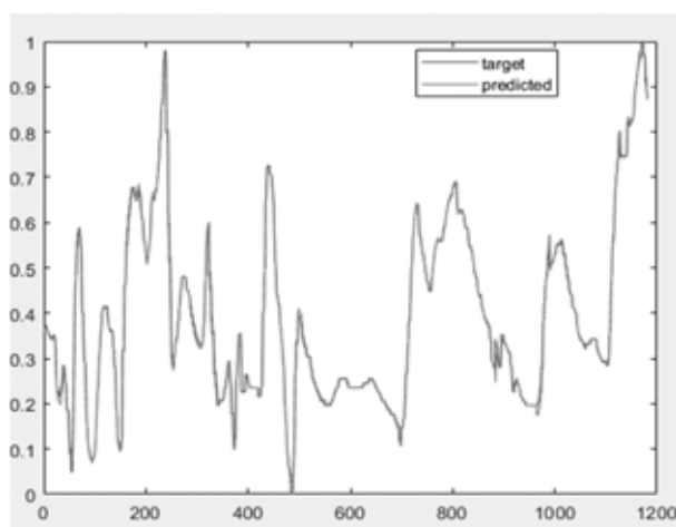
Рисунок 5. Сравнение ожидаемых и предсказанных нейросетью выходных значений сети LSTM
