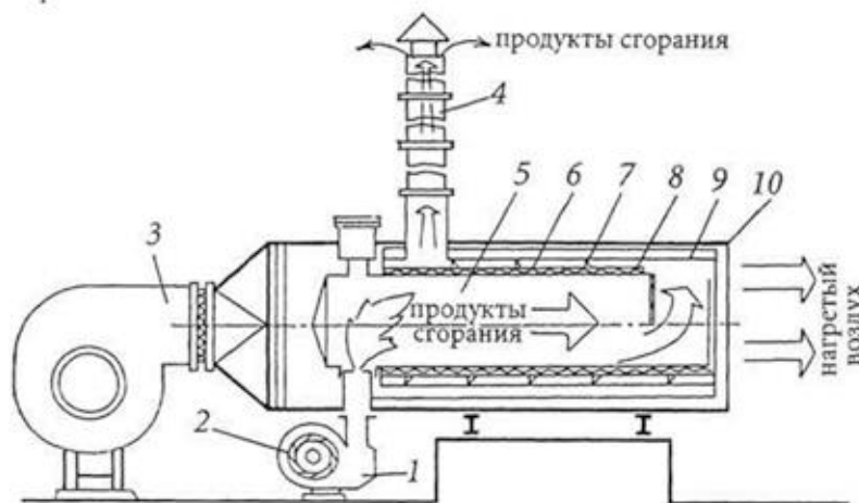
Рисунок 1 – Схема прямоточного (рециркуляционного) газозвоздушного теплообменника
