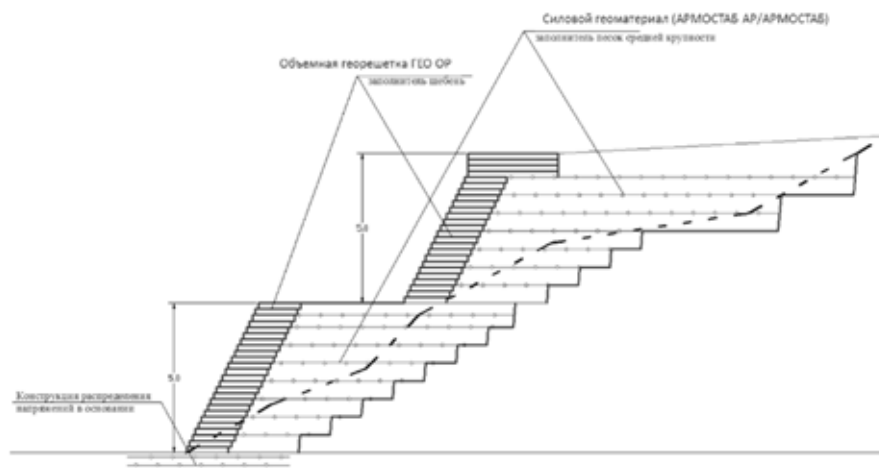
Рисунок 2 Подпорная стенка, армированная георешеткой
