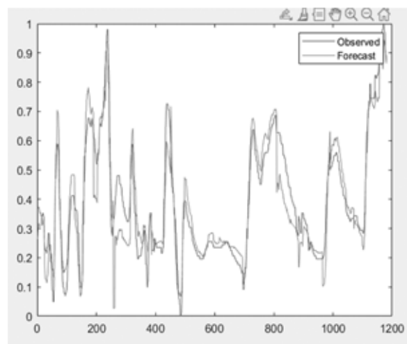
Рисунок 4. Сравнение ожидаемых и предсказанных нейросетью выходных значений многослойного перцептрона
