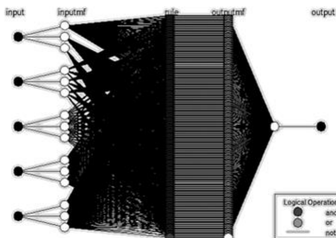
Рис. 3. Схема нечеткой нейронной сети
