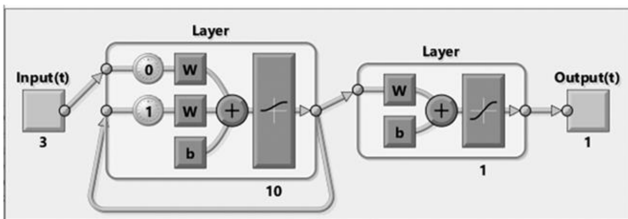
Рисунок 3. Модель нейронной сети на базе рекуррентной сети
