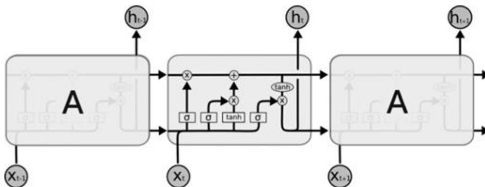
Рисунок 1. Повторяющийся модель в LSTM сети состоит из четырех взаимодействующих слоев
